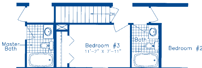
OPTIONAL BASEMENT PLAN
